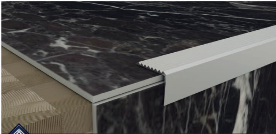
40x20 Tırtıklı Merdiven Basamak Profili /40x20 Stair Nosing Profile Ürün Kodu / Code : i240
