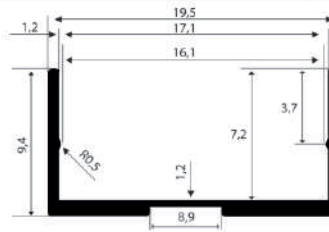
Ürün Teknik Bilgileri Product Technical Drawing
