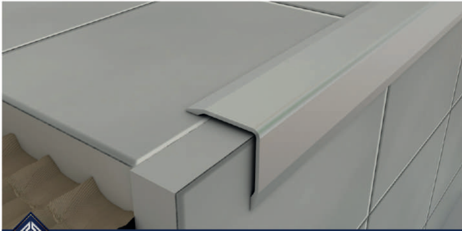
20x20 Alüminyum Köşe Profili / 20x20 Aluminium Corner Profiles Ürün Kodu / Code : i230
